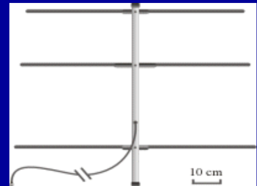
Antenne directionnelle Yagi
